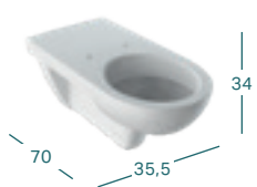
GEBERIT SELNOVA COMFORT SEINAPEALNE WC-POTT, PIKENDATUD VÄLJAU LATUVUS
