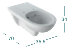
GEBERIT SELNOVA COMFORT SEINAPEALNE WC-POTT, PIKENDATUD VÄLJAU LATUVUS, RIMFREE
